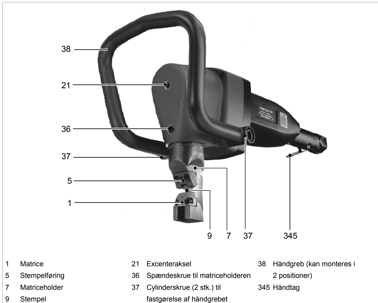
Nibler TruTool N 700
